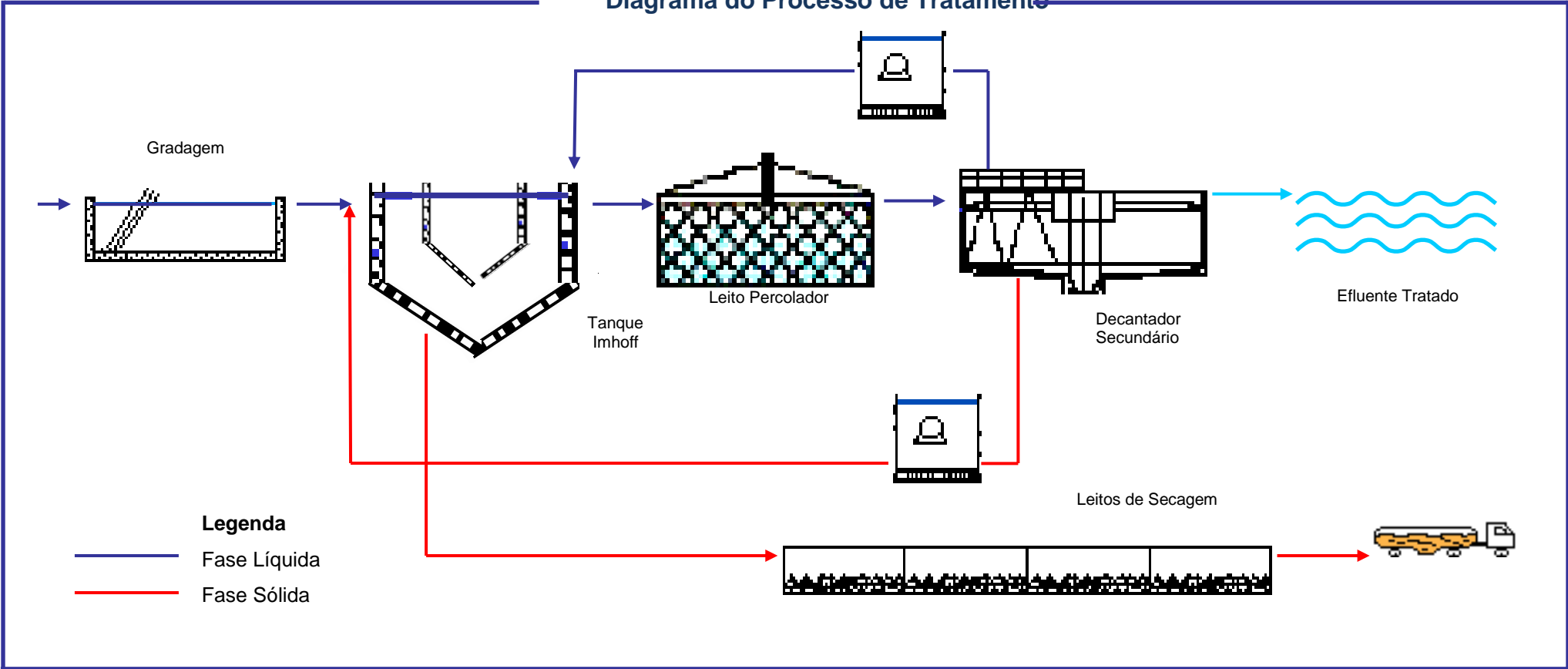
Diagrama do Processo de Tratamento
